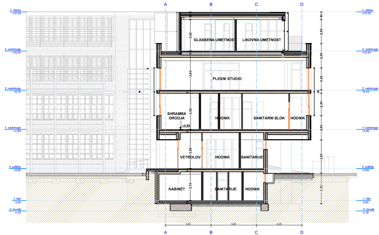
2-3 prečni prerez
