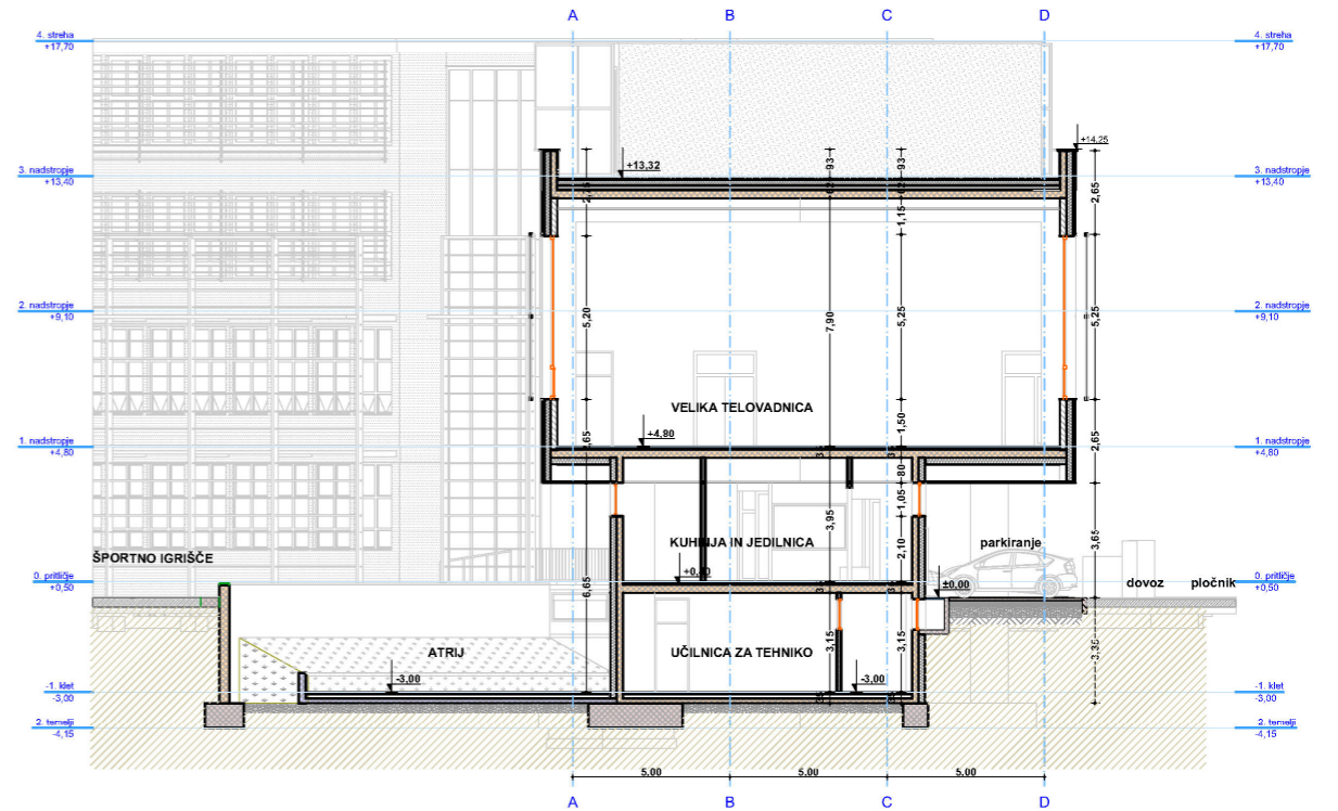
7-8 prečni prerez
